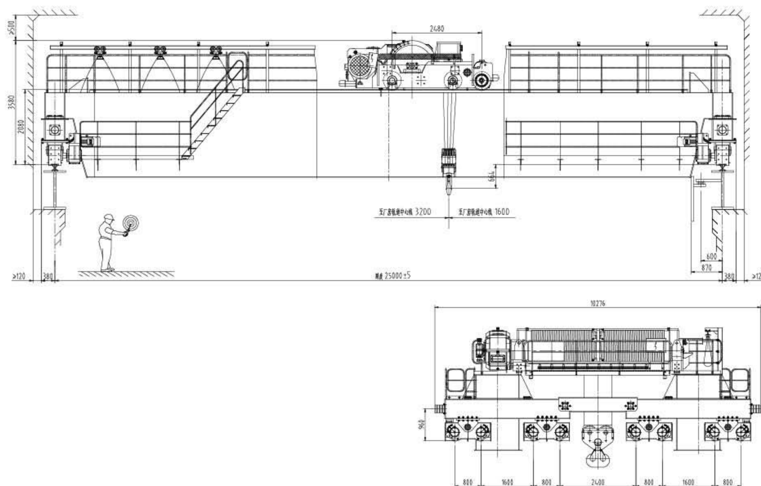
载荷 Capacity 320t 跨度 Span 25m 起升高度 Max Lifting Height 20m 起升速度 Lifting Speed 主钩0-1.2变频 Main Hook 0-1.2 VVVF 小车速度 Cross Traveling Speed 20/5 m/min变频 VVVF 大车速度 Long Traveling Speed 40/10 m/min变频 VVVF 起升电机功率 Lifting Motor Power 主钩 Main Hook 75kW 小车运行电机功率 Crossing Traveling Motor Power 2 × 15KW 大车运行电机功率 Long Traveling Motor Power 4 × 15KW 小车自重 Trolley Dead Weight 40.3t 桥架重量 Bridge Dead Weight 105t 供电电压 Power Source 380V/48V/50Hz 起重机工作级别 Crane Woking Class FEM A5 小车运行 Cross Traveling FEM 2m(M5) 大车运行 Long Traveling FEM 2m(M5) 整机功率 Total Power 165kW 最大轮压 Max. Wheel Loading 526KN
